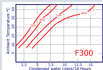
KONDENSOWANA WODA PRZY RÓŻNYCH TEMPERATURACH I WILGOTNOŚCI WZGLĘDNEJ
