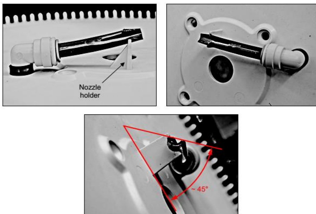
Rys. 4.5 Pozycjonowanie dyszy
